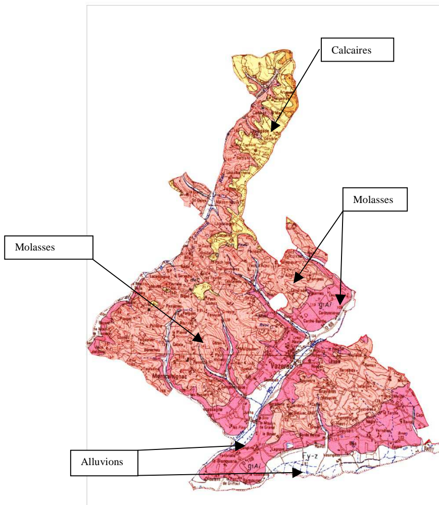
Figure 5 : Carte géologique de Vazerac - Extrait de la carte géologique du BRGM
